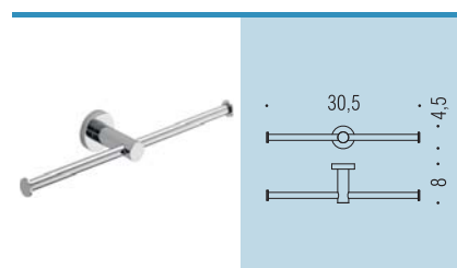
W4990 Porta rotolo doppio Double Paper holder
